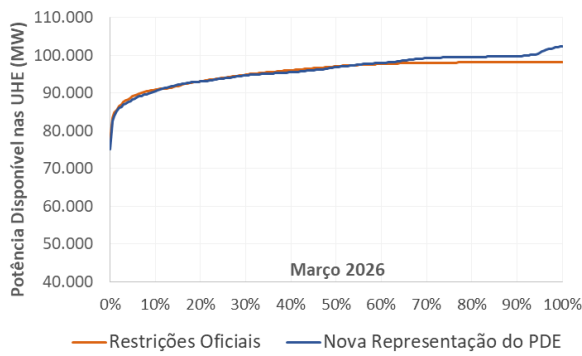
Gráfico 3 - 36: Potência Disponível – Usinas Hidrelétricas – SIN – março/2026
