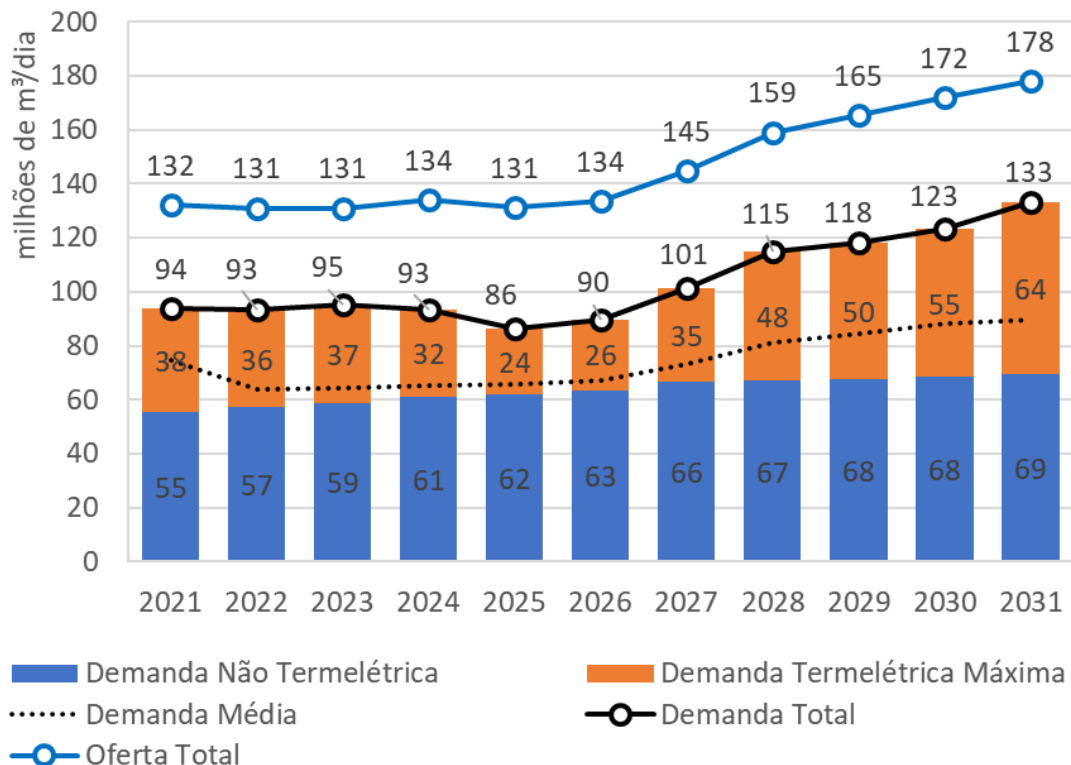
Gráfico 7 - 6: Balanço de gás natural da Malha Integrada do Brasil
