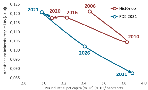
Gráfico 2 - 4: Sendero energético industrial
