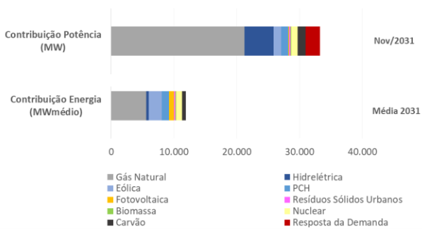
Gráfico 3 - 31: Contribuição de Energia e Potência da Expansão de Referência do PDE 2031
