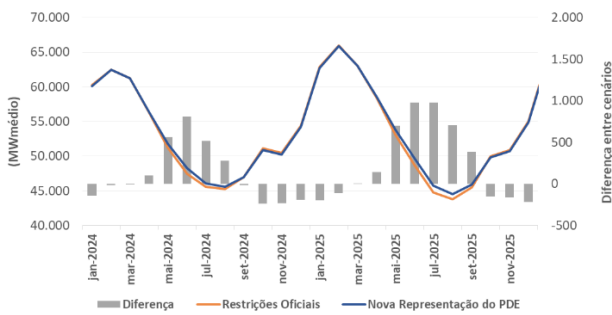
Gráfico 3 - 8: Geração Hidrelétrica no SIN com e sem novas restrições operativas
