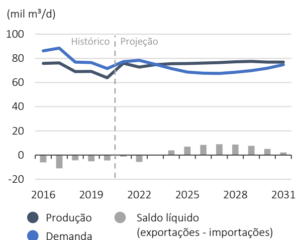
Gráfico 6 - 7: Balanço nacional de gasolina A
