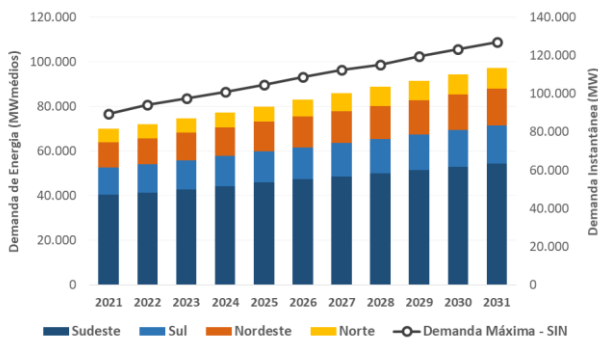
Gráfico 3 - 4: Oferta termelétrica retirada do Caso Base do PDE 2031
