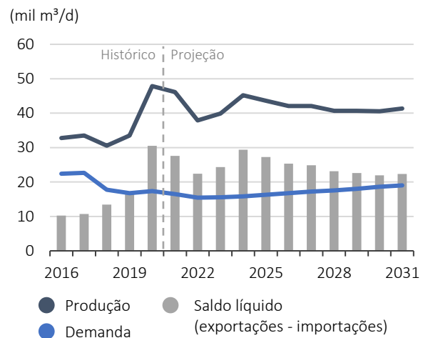
Gráfico 6 - 11: Balanço nacional de óleo combustível
