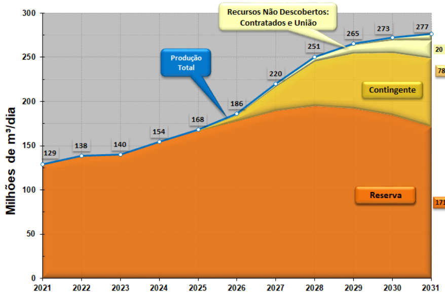
Gráfico 5 - 3: Previsão da produção bruta diária de gás natural nacional
