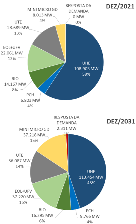
Gráfico 3 - 32: Configuração do Cenário de Referência do PDE 2031 em 2021 e 2031
