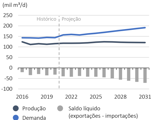
Gráfico 6 - 10: Balanço nacional de óleo diesel A
