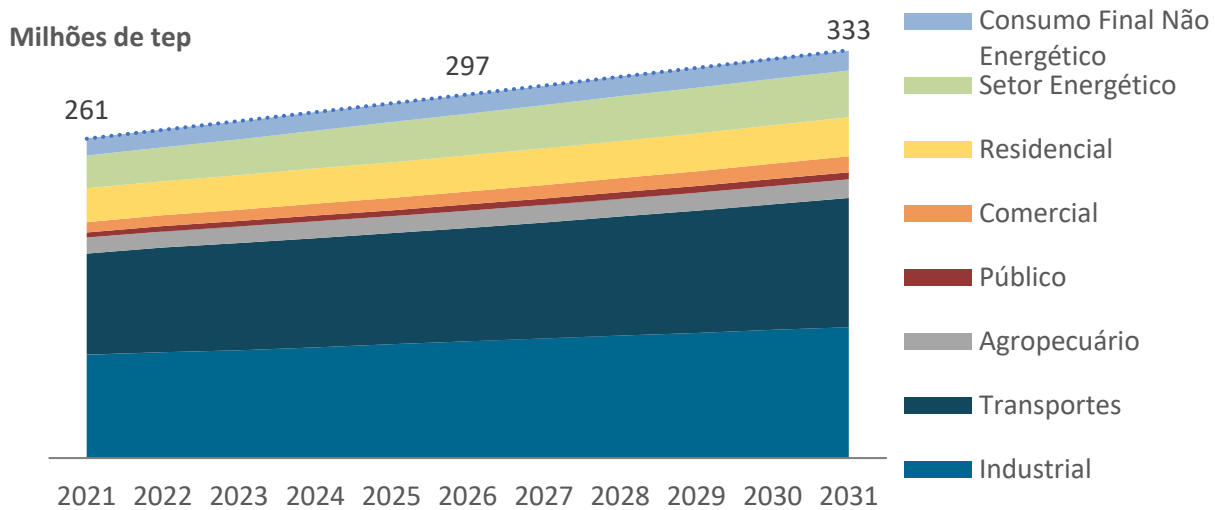
Gráfico 2 - 1: Consumo final de energia por setor
