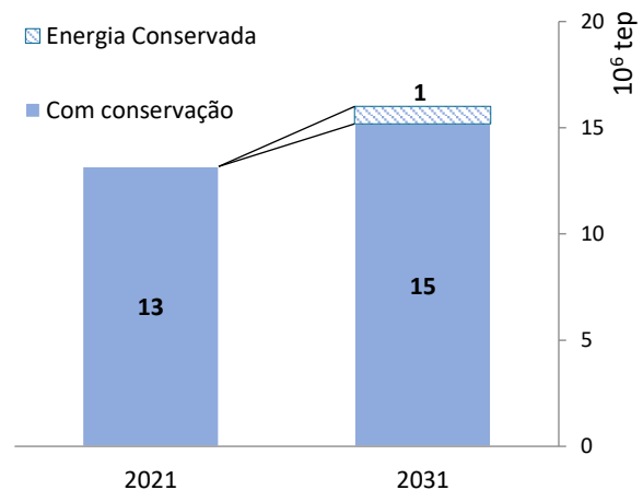
Gráfico 9 - 16: Setor agropecuário: Consumo de energia total e eficiência energética
