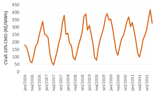
Gráfico 3 - 40: Atendimento ao Critério de Suprimento de Energia
