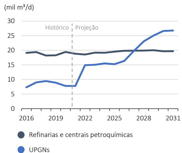
Gráfico 6 - 5: Produção nacional de GLP por tipo de unidade produtora
