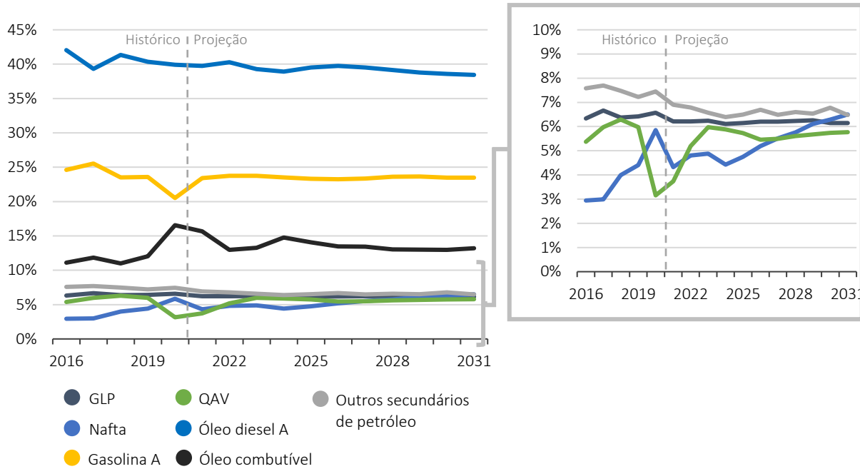
Gráfico 6 - 4: Perfil de produção das refinarias nacionais (%)
