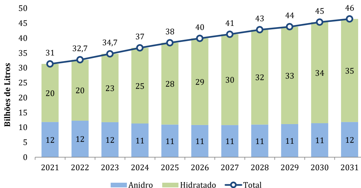
Gráfico 8 - 4: Projeção da oferta total de etanol
