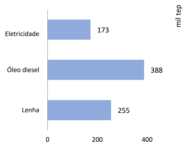
Gráfico 9 - 15: Setor agropecuário: Ganhos de eficiência por fonte em 2031 (mil tep)
